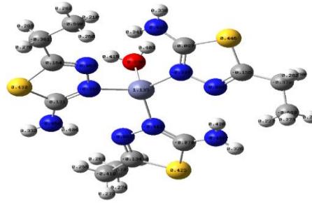
10-rasm. Akva-tris(2-amino-5-etil-1,3,4-tiazol)-Rux (II) dinitrat ( [\text{Zn}(\text{C}_4\text{H}_7\text{N}_3\text{S}_2)_3(\text{OH}_2)](\text{NO}_3)_2 ) molekulasida elektron zaryadlarning taqsimlanishi
