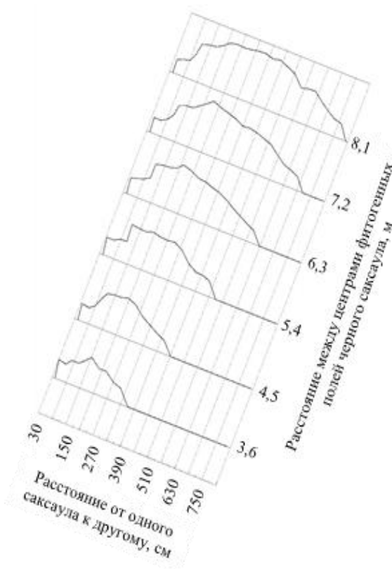
Рис. 3. Продукция надземной фитомассы (г/м 2 в воздушно-сухом весе) мятлика луковичного в зависимости от удаленности особей черного саксаула друг от друга.
