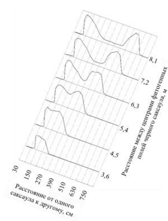
Рис. 2. Годичный прирост надземной фитомассы (г/м 2 в воздушно-сухом весе) полыни раскидистой в зависимости от удаленности особей черного саксаула друг от друга.
