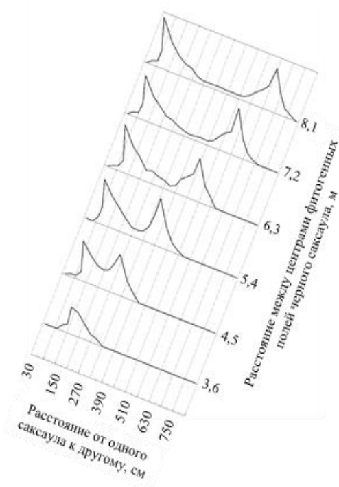
Рис. 5. Продукция надземной фитомассы (г/м 2 в воздушно-сухом весе) разнотравья в зависимости от удаленности особей черного саксаула друг от друга.
