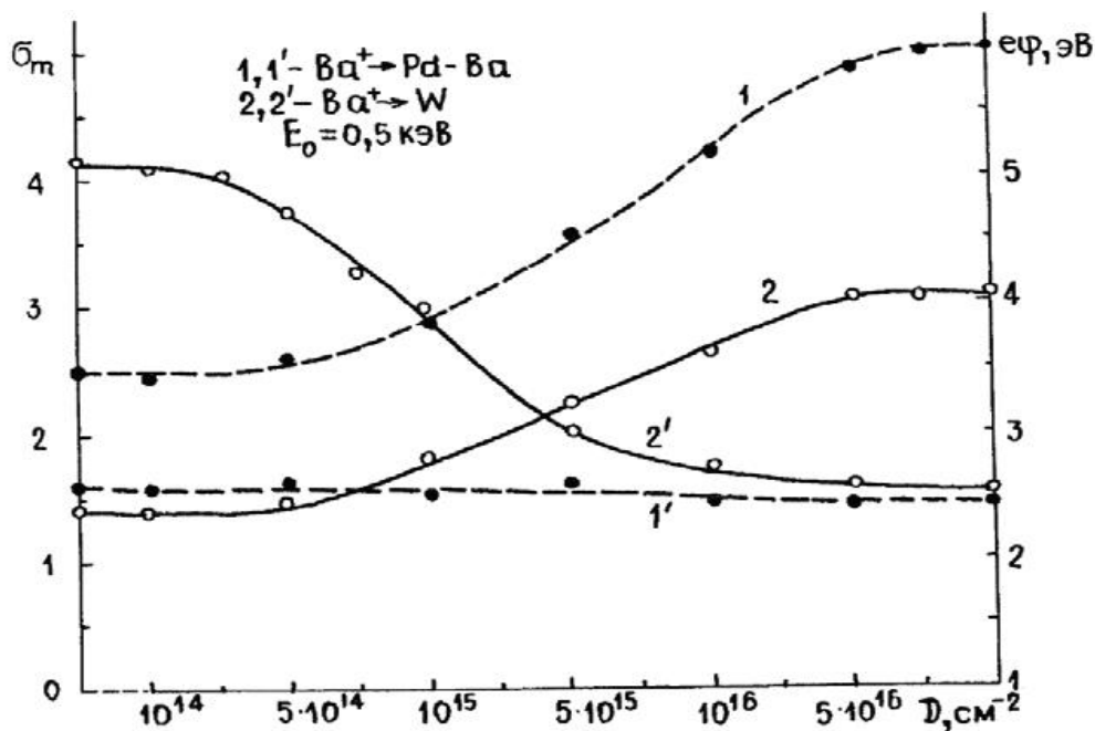
Зависимости \sigma_m (1 и 2) и e\varphi (1' и 2') от дозы облучения для Pd-Wa и W, легированных ионами \text{Ba}^+ с E_0 = 0,5 \text{ кэВ} .
