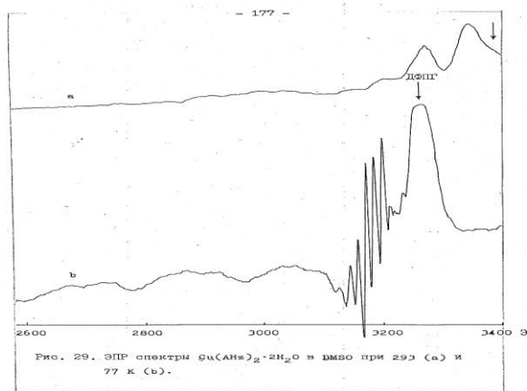
ЭПР-спектры \text{Cu}(\text{АНз})_2 \cdot 2\text{H}_2\text{O} в DMSO при 293 (а) и 77 К (б).
