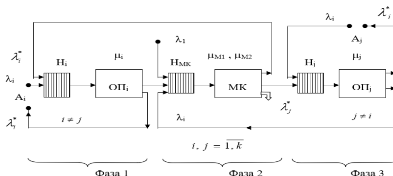
Рис.1. Фрагмент взаимодействия двух любых абонентов: «абонента A_i и абонента A_j, i \neq j .
