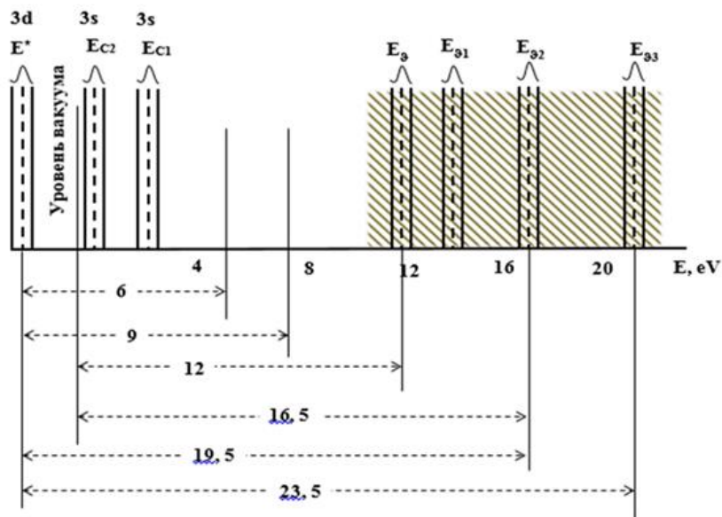
Построение энергетической диаграммы плёнки SiO_2 на кремний.
