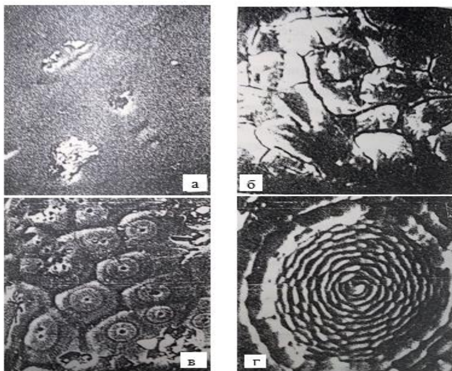
Микрофотографии поверхности: аморфной пленки \text{SiO}_2 – а; пленки \text{SiO}_2 , легированной ионами \text{Ba}^+ , E_0 = 0,5\text{эВ} при \Phi = 4 \cdot 10^{14} \text{ см}^{-2} – б; пленки \text{SiO}_2 , легированной барием при \Phi = 6 \cdot 10^{16} \text{ см}^{-2} – в; г – участок кристаллизованной области.
