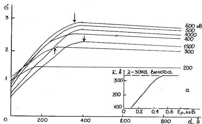
Зависимости \sigma от толщины d плёнок \text{SiO}_2 , осажденных на поверхности \text{Si} для разных энергий первичных электронов. \lambda'(E_p) – зависимость глубины выхода ИВЭ от энергии электронов для \text{SiO}_2 .
