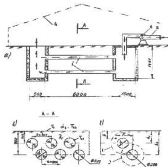
Рис. 3. Грунтовой подпочвенный аккумулятор тепла (а) и расчетные схе-мы теплопередачи ряда труб (б) и температурного поля вокруг двухтрубного теплопровода (в) в грунте гелиотеплицы: 1-чугунные теплоаккумулирующие трубы ( d = 200 мм); 2-вентилятор; 3-канал для подачи отходящих дымовых газов; 4-
