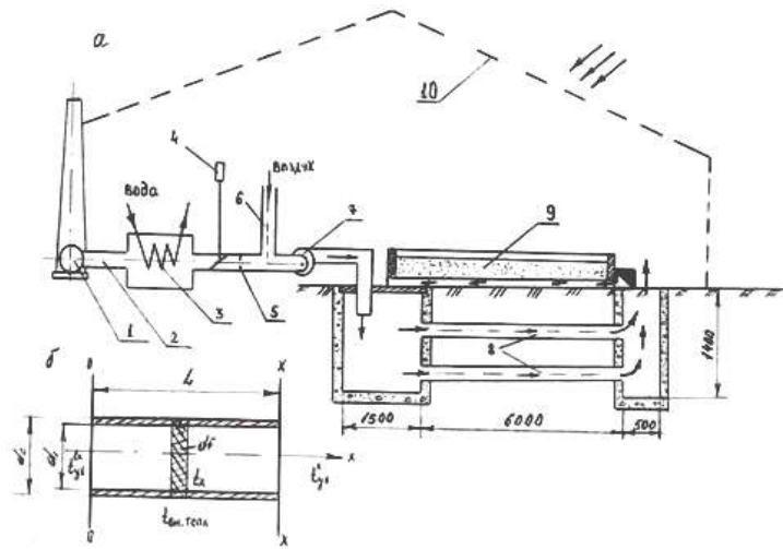
Рис. 2. Принципиальная схема использования отходного тепла для отоп-ления теплиц и обогащения воздуха в нем диоксидом углерода (а) и расчетная тепловая схема вытяжного дымохода круглого сечения (б): 1-котел; 2-газовый канал; 3- водяной теплообменник; 4-сервомотор с запорным клапаном; 5-ограни-чительная диафрагма; 6-канал для подсоса воздуха; 7-центробежный вентилятор.
