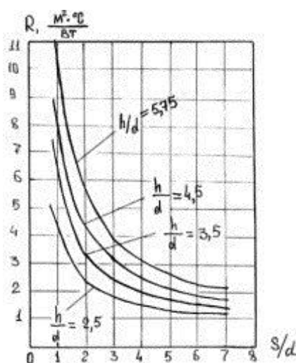
Рис. 4. Термические сопротивления тепличной почвы при передаче тепла от одной из ряда труб, находящихся на различной глубине в грунте гелиотеплицы.
