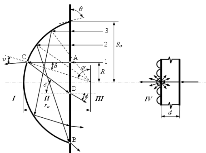
Рис. 1. Модель капли конденсата: 1 - типичный случай однократного отражения, 2 - предельный случай однократного отражения, 3 - типичный случай двух и более кратного отражения; I - воздух, II - вода, III - стекло, IV – прозрачный слой с капельным конденсатом.
