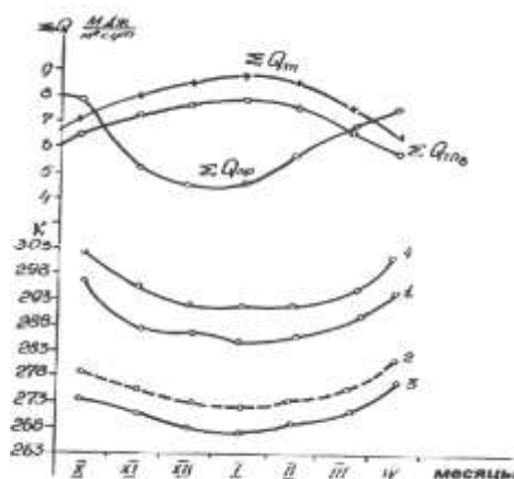
Рис.1. Характеристики внешних воздействий и изменение теплопотерь гелиотеплицы для отопительного периода по многолетним данным (1988-1997 гг.). \Sigma Q_{np} - солнечная радиация, прошедшая внутрь теплицы; \Sigma Q_{ТПВ} , \Sigma Q_{np} - потери тепла в случае аккумуляирования и без аккумуляирования тепла солнечной энергии: 1-температура воздуха внутри теплицы; 2, 3-средняя и минимальная температуры наружного воздуха; 4- температура субстрата – грунта теплицы на глубине 15 см от поверхности.
