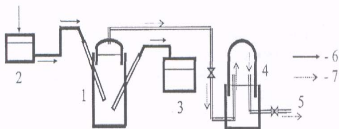
1-расм. Оддий биогазгенераторли курилманинг схемаси: 1-биогаз генератор – метантэнк; 2-биомассани қабул қилиш курилмаси; 3-қайта ишланган маҳсулотларни тўплаш мосламаси; 4-сувли газголдер; 5-истеъмолчи учун ажратилган биогазнинг чиқиш йўлаги; 6-биомасса; 7-биогаз.
