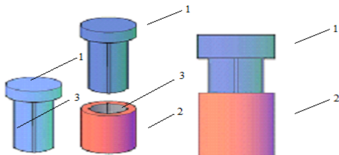
4-расм. Пуансон ва ҳалқанинг боғланиши: 1-пуансон; 2-ҳалқа; 3-шлица.
