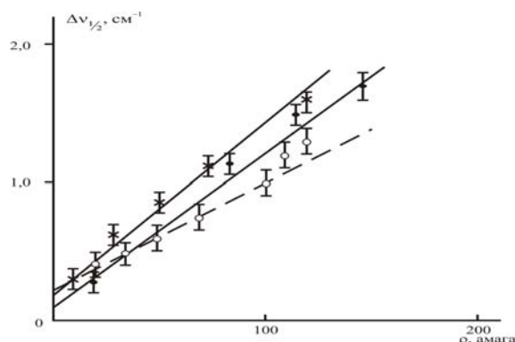
Рис. 1. Зависимость полуширины полосы \nu_1 \text{CH}_4 от плотности при T = 295 \text{ K} . \bullet - чистый метан, \circ - смесь с Ar, * - смесь с Kr.
