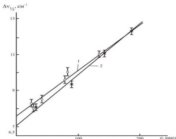
Рис. 2. Зависимость от плотности полуширины полосы \nu_1 \text{CD}_4 в смеси с аргоном 1— \circ - 295 K, 2 — * - 200 K.
