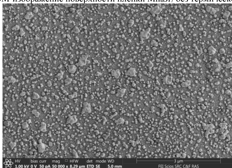
Рис. 4. РЭМ-изображение поверхности пленки Mn_4Si_7 после термического отжига.
