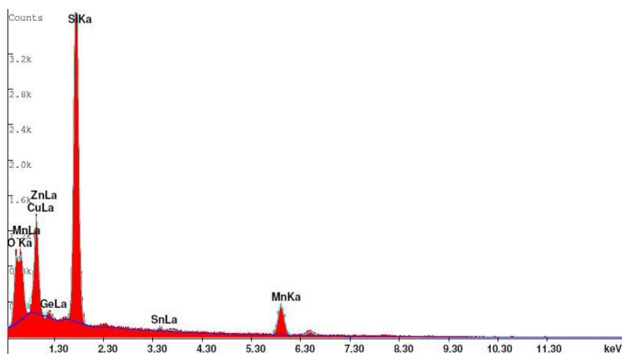
Рис. 5. Рентгеновский спектр пленки Mn_4Si_7 .
