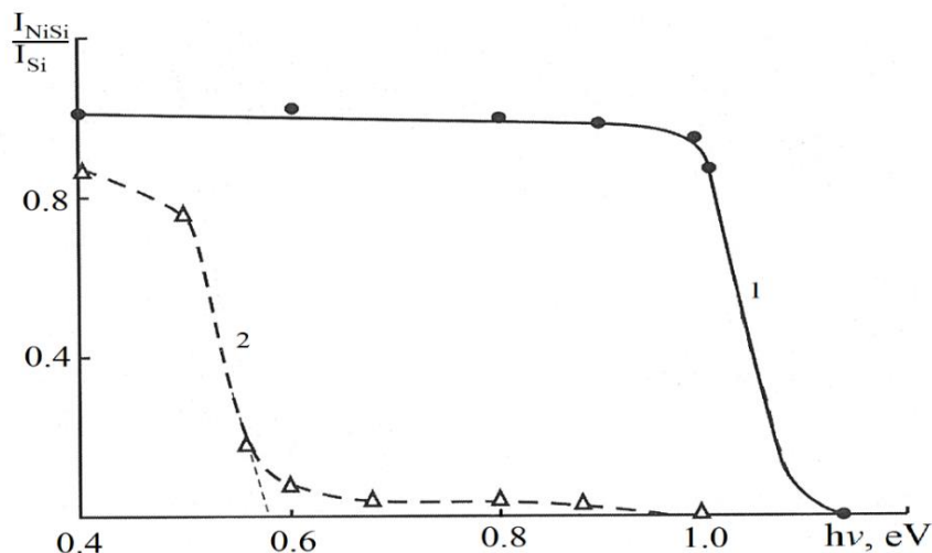
Рис. 3. Зависимость интенсивности проходящего света от энергии фотонов для 1- чистого Si(111); 2-системы Si/NiSi 2 /Si (111). d_{NiSi_2} = 20 нм, d_{Si} = 50 нм.
