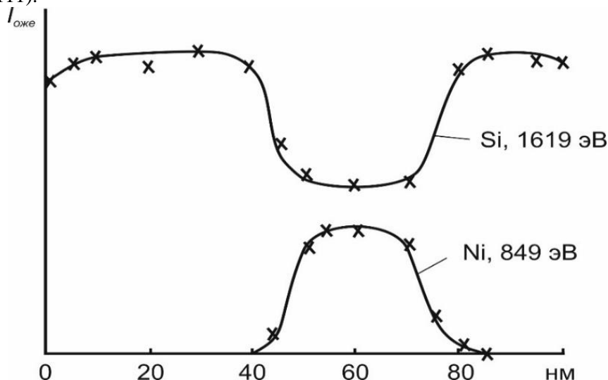
Рис.2. Зависимость интенсивности Оже пиков Si (E=1619 эВ) и Ni (E=848 эВ) для системы Si/NiSi 2 /Si(111); d_{Si} = 50 \text{ нм} , d_{NiSi_2} = 20 \text{ нм}
