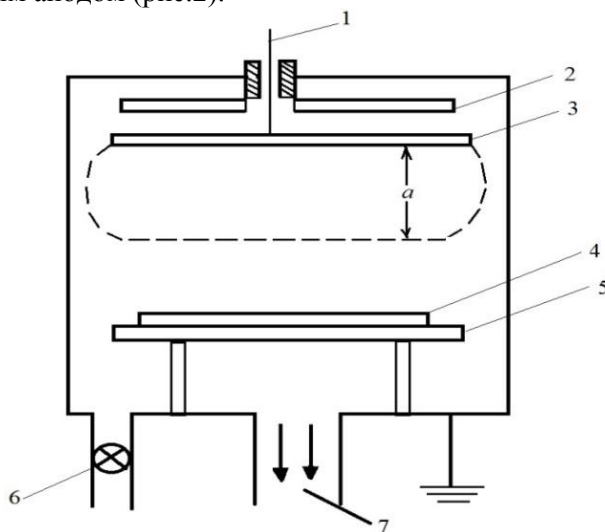
Рис. 2. Схема устройства катодного распыления диодного типа:
