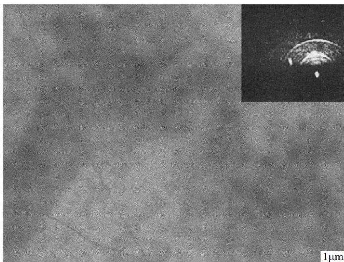
Рис. 1. РЭМ- и ДБЭ (вставка) изображения поверхности системы Si/NiSi 2 /Si(111). Пленки Si напылялась при T≈1000 К с толщиной ~50 нм.
