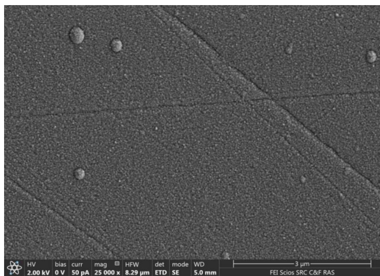
Рис. 3. РЭМ-изображение поверхности пленки Mn_4Si_7 без термического отжига.
